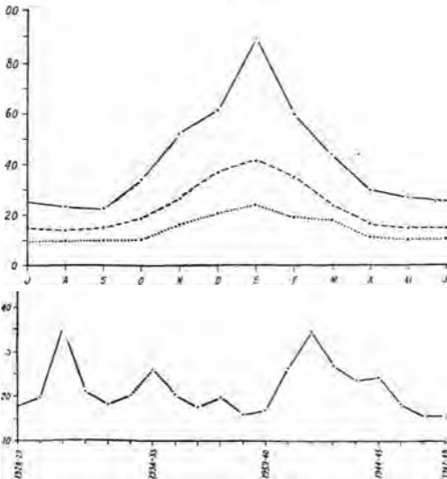
FIG. 136 — Curvas de caudales del río Atuel, medias mensuales y anuales.
