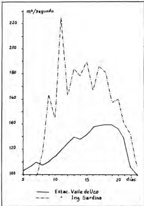
Fig. 156 - Curva de caudales máximos correspondientes a la crecida de diciembre de 1953, según R. O. Barrera.
