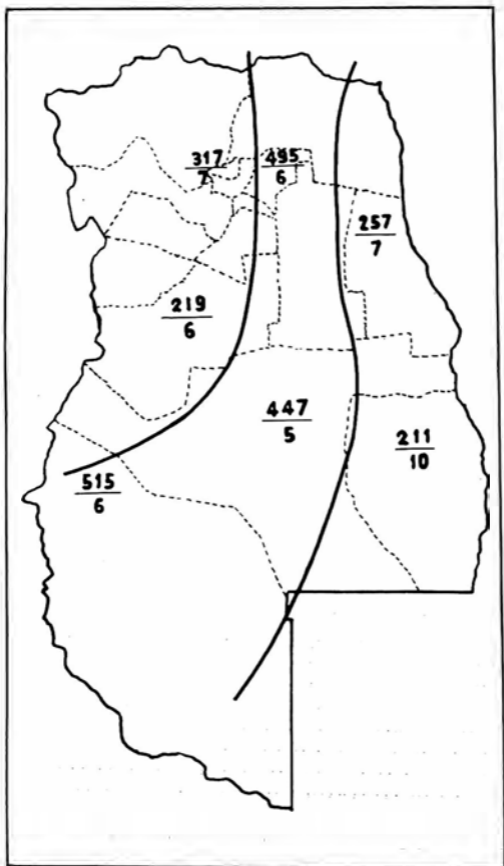
FIG. 170 — Frecuencia y velocidad media del viento.
