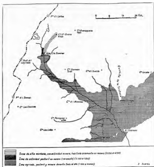
FIG. 137 - Bosquejo de actividades humanas en el valle del Atuel.
