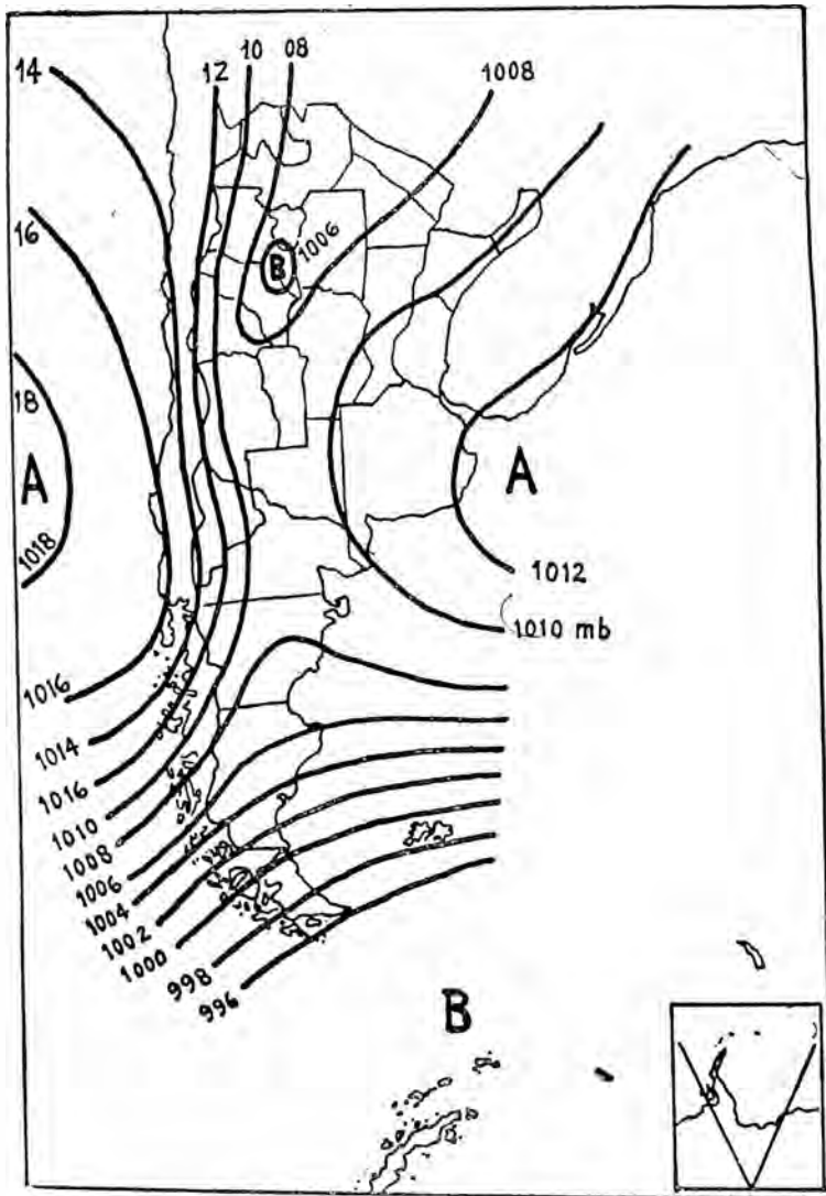
FIG. 3 — Presión atmosférica media, al nivel del mar (1901-50), en enero, según K. Wolken.
