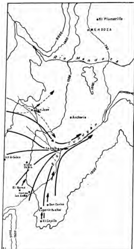
FIG 195 — Líneas de corrientes en superficie, según J. G. Edinger.
