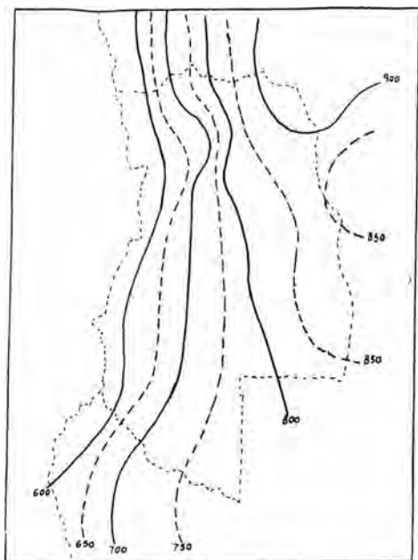
FIG. 145 — Evapotranspiración potencial, según F. Albany.
