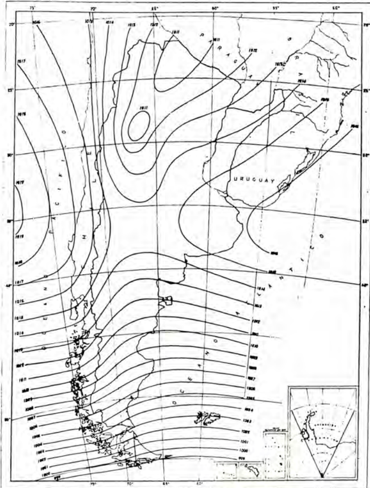
FIG. 2 — Presión media anual, según el Atlas Climático de la República Argentina, del Servicio Meteorológico Nacional, 1960.
