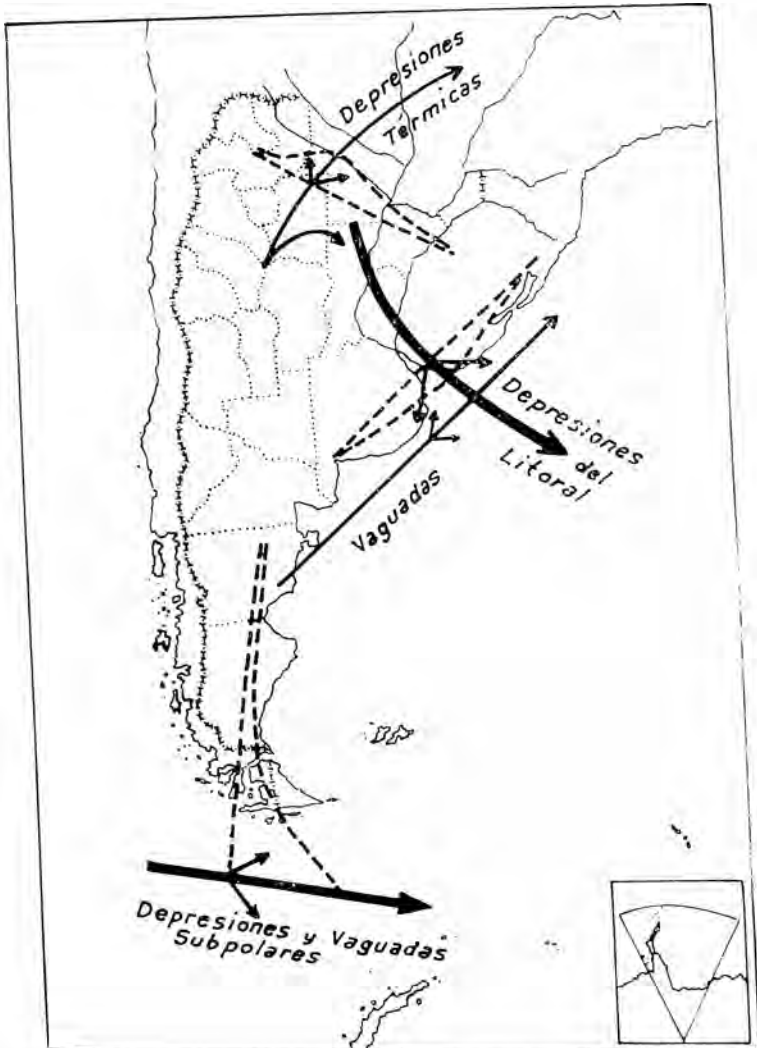
Fig. 9 — Trayectorias de los centros de las depresiones. Invierno (junio a agosto), según K. Wolcken.
