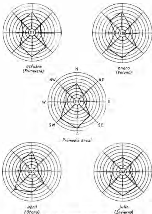
FIG. 199 — Vientos en San Carlos.
