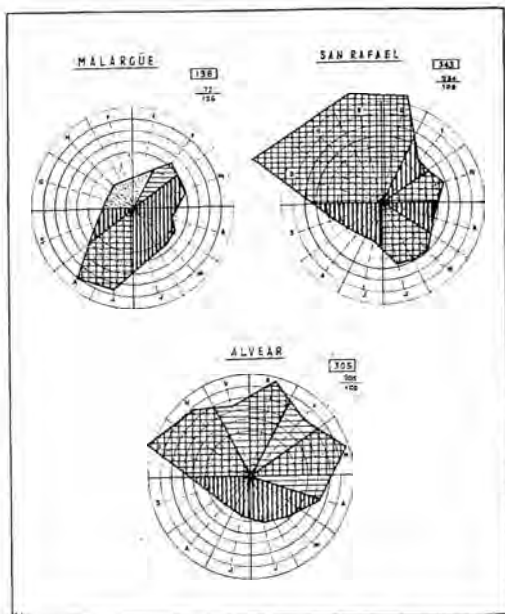
FIG. 153 — Precipitaciones correspondientes a Malargüe, San Rafael y General Alvear.
