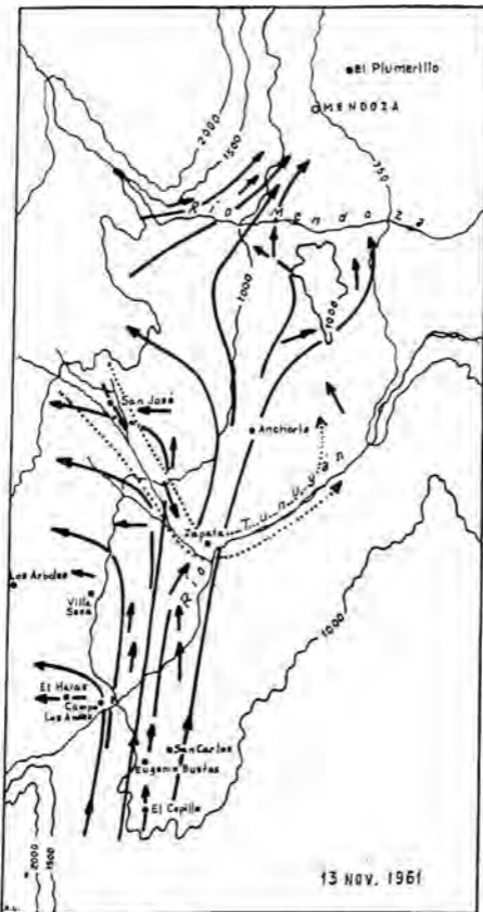
Fig. 193 - Líneas de corrientes en superficie, en la depresión de San Carlos según J. G. Edinger.
