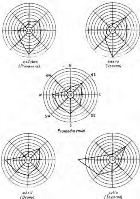
Fig. 179 — Vientos, según datos del Observatorio Regional Mendoza.
