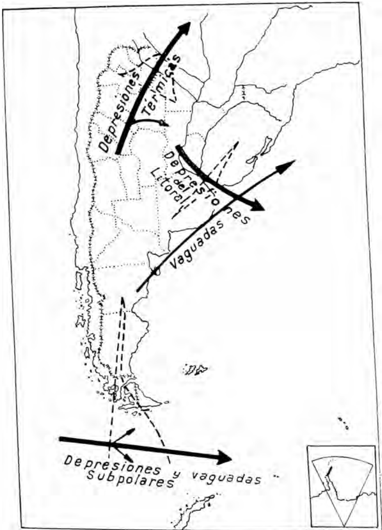
FIG. 10 - Trayectorias de los centros de las depresiones. Verano (diciembre a febrero), según K. Wolken.
