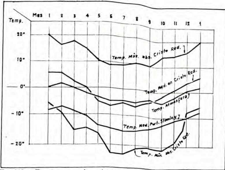
FIG. 120 — Temperatura media, máxima y mínima absoluta y de la atmósfera libre en Cristo Redentor y temperatura media de Port Stanley, según K. Pietrzykowski.
