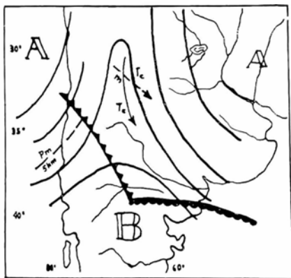
FIG. 171 — Situación típica de Zonda, según W. Georgii.
