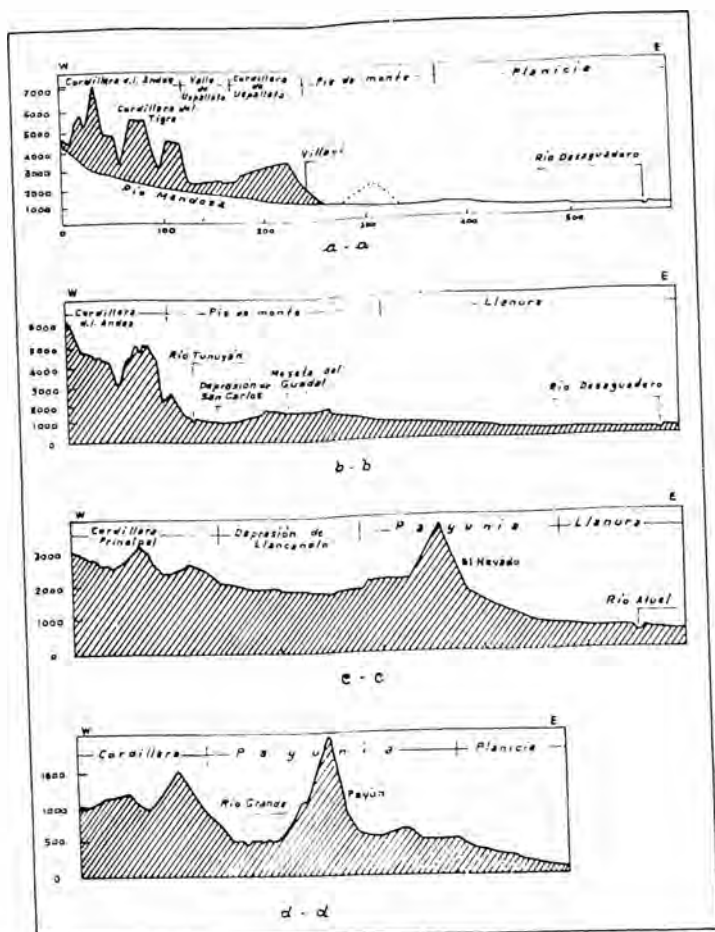
FIG. 119 — Perfiles topográficos correspondientes al bosquejo geomorfológico (Fig. 118).
