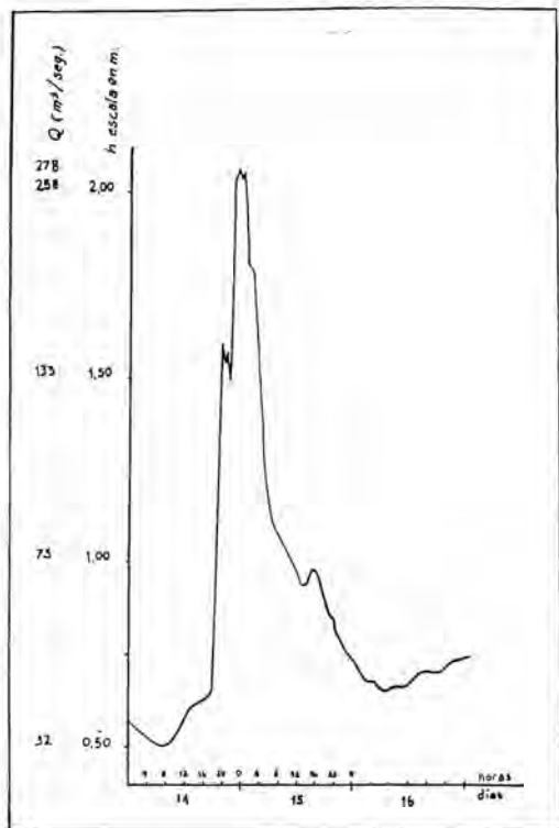
FIG. 157. — Registro del limnigrafo en la estación Ing. Sardina, durante la crecida extraordinaria de diciembre de 1962, según R. O. Barrera.
