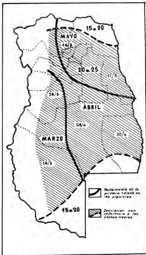
Fig. 168 — Comienzo de las heladas y desviación probable respecto de las fechas medias.
