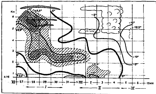
FIG. 174 -- Desarrollo de un período de Zonda, de acuerdo con sucesivas ascensiones en avión, según W. Georgii.
