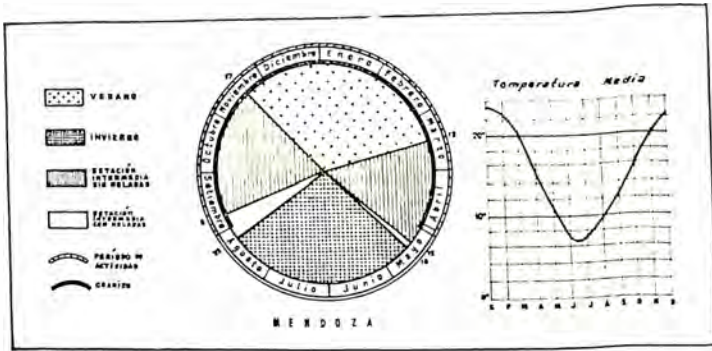
FIG. 11 — Comparación de las estaciones térmicas, períodos de heladas, granizo y actividad correspondiente a Mendoza.
