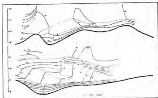
FIG. 192 — Corte vertical del campo térmico vertical de la depresión de San Carlos, según J. G. Edinger.
