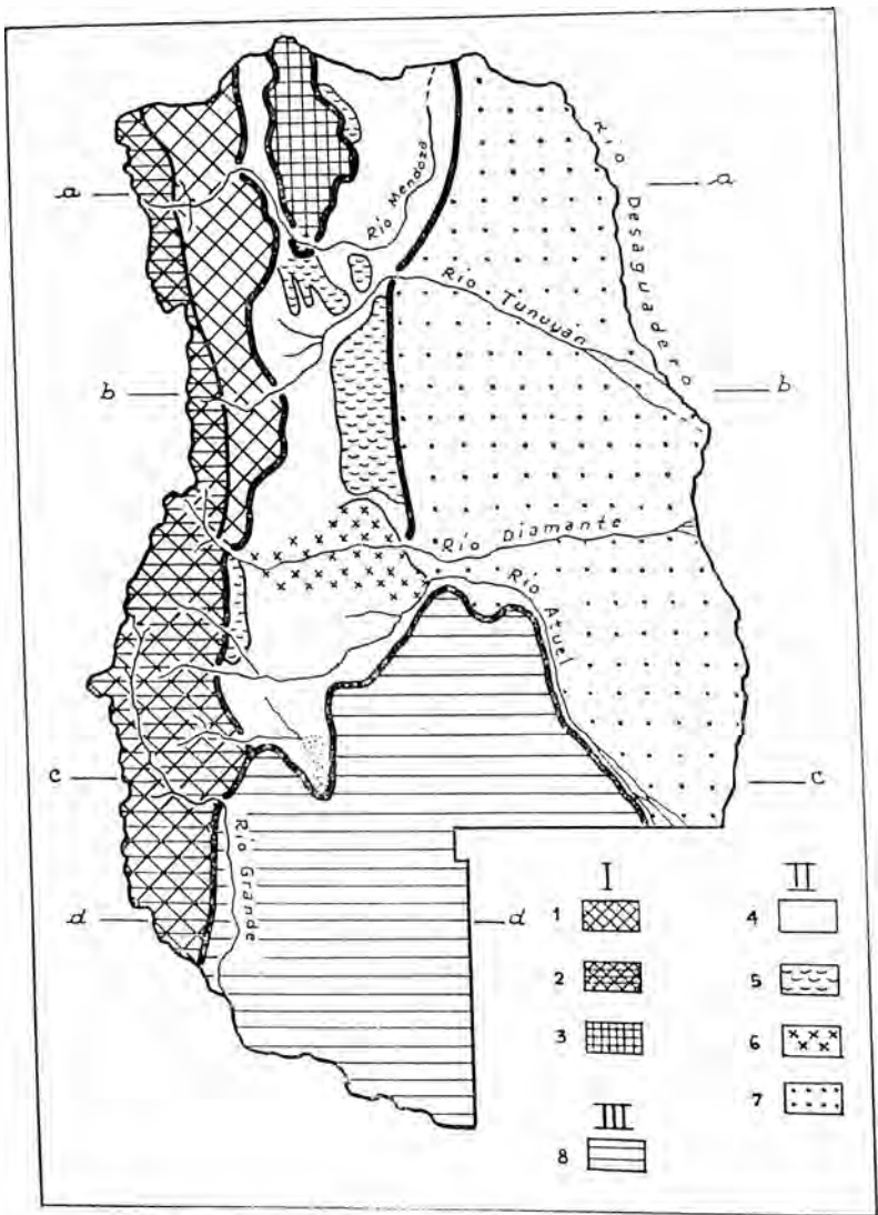
Fig. 118 — Bosquejo geomorfológico. I) Región de las montañas: 1) cordillera principal; 2) cordillera frontal, y 3) precordillera. II) Región de las planicies: a) piedemonte: 4) depresiones y valles; 5) bad-lands (huayquerías), y 6) macizo antiguo de San Rafael; b) 7) llanura, III) Región volcánica, de la Payunia.
