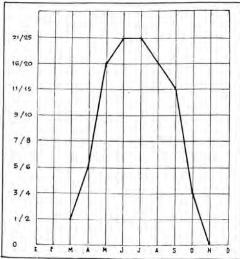
FIG. 190 — Frecuencia media de heladas en San Carlos.
