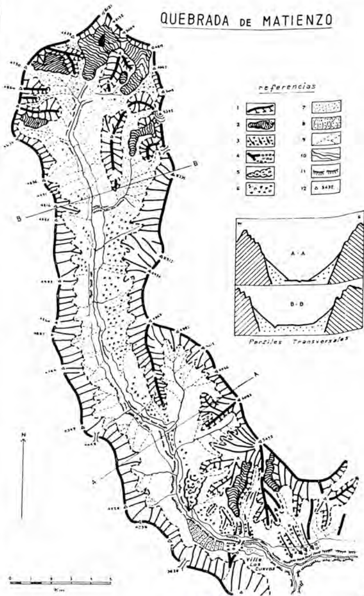
FIG. 124 — Bosquejo geomorfológico de la quebrada de Matienzo: 1) paredes rocosas, afloramientos y circos glaciares; 2) glaciares; 3) derrumbes; 4) corredores de avalanchas; 5) coladas de piedras y barro; 6) campos de piedras; 7) sedimentos fluvioglaciares; 8) depósitos de soliflucción o varves; 9) cursos temporarios sobre lechos de piedras (ríos de piedras); 10) lechos fluviales, ríos y arroyos permanentes; 11) depósitos de vertientes y aluviales terrazados, y 12) cumbres y cotas.
