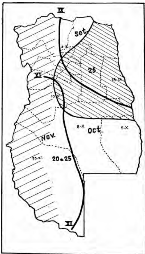
Fig. 169 - Fecha media de terminación de las heladas y desviación probable.
