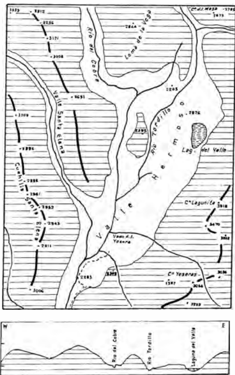
Fig. 130 - Bosquejo geomorfológico de valle Hermoso.
