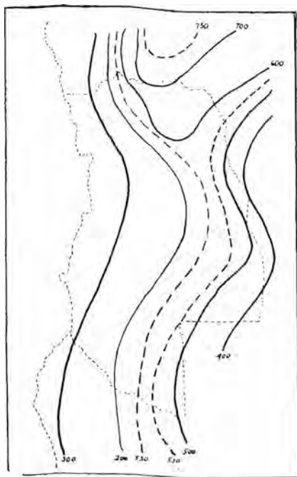
Fig. 146 - Deficiencia de agua (promedio anual), en mm.
