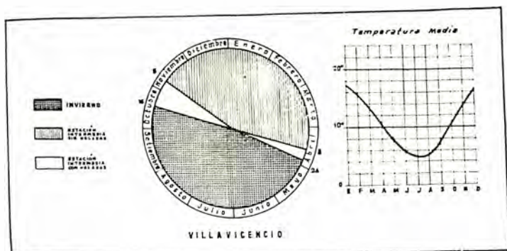
FIG. 12 — Comparación de las estaciones térmicas, períodos de heladas, granizo y actividad, correspondiente a Villavicencio.
