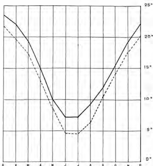
FIG. 205 — Temperaturas medias: — Mendoza — — — Malargüe.
