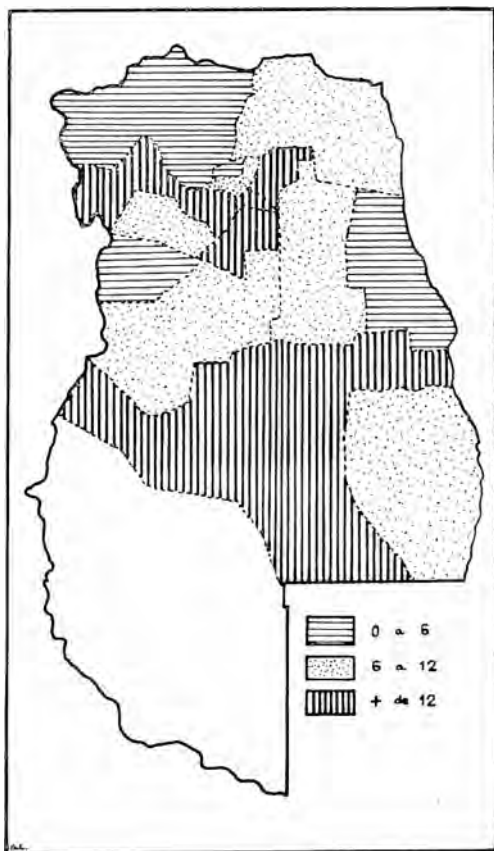
FIG. 166 – Número de granizadas por departamentos.
