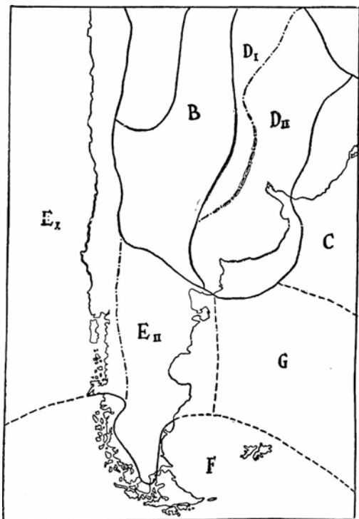
FIG. 150 - Regímenes de precipitaciones, según J. Prohaska. B. Régimen subtropical continental durante todo el año. D I. Régimen de transición. E I y II. Régimen subtropical pacífico en verano y de la zona templada en invierno.
