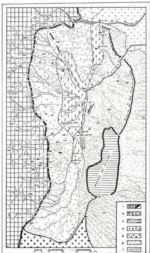
FIG. 186 — Bosquejo geomorfológico de la depresión de San Carlos: 1) montaña; 2) unidad compleja (glacis superior y principal, con conglomerados de Mogotes; 3) glacis de las Huayquerías; 4) playa y cultivos; 5) bloque elevada del Diamante; 6) playas del oasis del norte, y 7) médanos.
