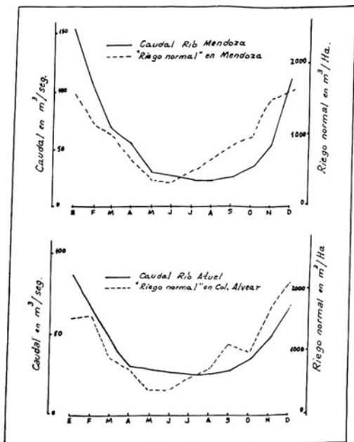
FIG. 159 — Relaciones entre riego normal y caudales del río Mendoza y Atuel, según J. Papadakis.
